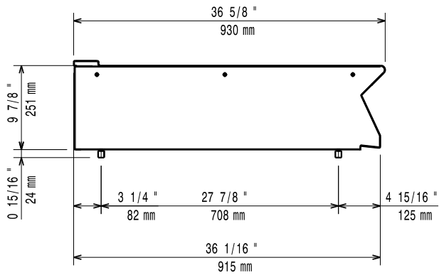
俯视
